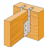
Bevestiging van een bretelbeugel met N3.75
