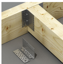
Bevestiging balk op balk
