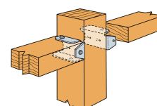
Bevestiging regel op kolom
